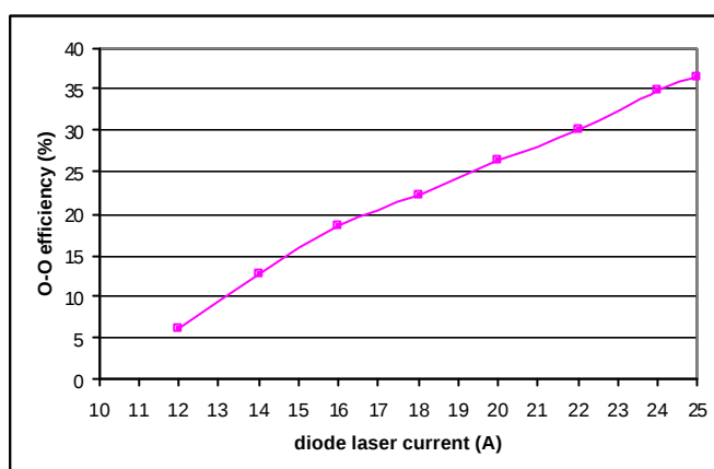
图 4 光光转换效率与驱动电流的关系 Fig. 4 0-0 conversion efficiency vs driving current
