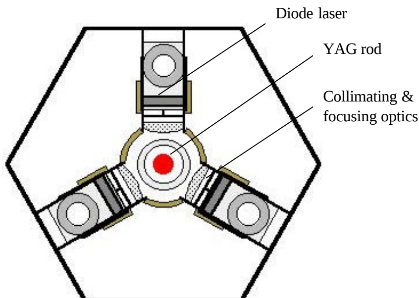
图 2 侧面泵浦结构
