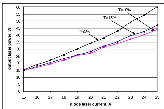
图 3 Nd:YAG 激光输出功率与驱动电流的关系 Fig. 3 Nd:YAG laser power vs driving current
